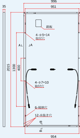
裏面図
